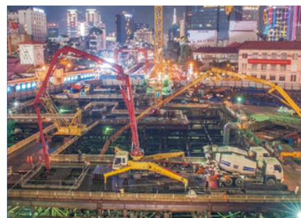
夜間にも行われたコンクリートの打設
